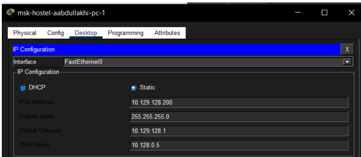
Рис. 2.14: Настройка IP-адреса на ПК сети общежития
